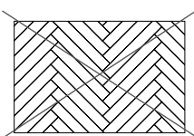
рисунок « колос» под углом 45° (не желательно)
