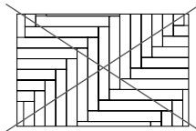
Pose en chevron 90° (déconseillé)
